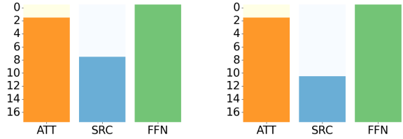
(a) Token: [Space]wollen (b) Token: struktur
